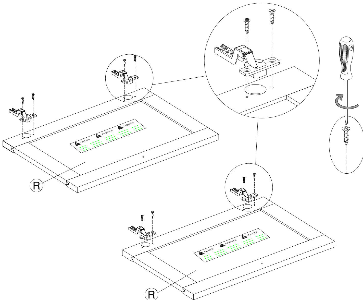
Hinge Arm
